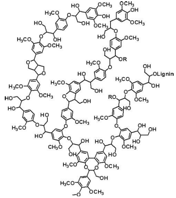
Lignin
